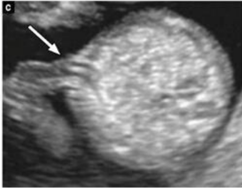
图6 胎儿腹部。腹部轴位水平显示腹围测量平面（虚线），显示胃（S）和脐静脉（UV）。（b）腹部冠状面显示肾盂中央呈低回声（K，箭头），胃（S）和膈肌（Diaph，线）。（C）脐带插入（箭头）。注意两条脐动脉是可见的。
